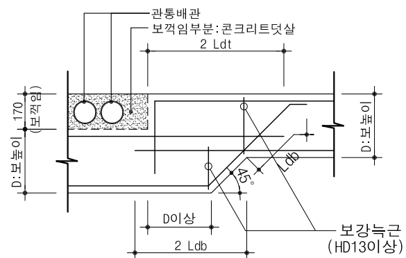
보격임 상세"A" - (2층바닥적용)
