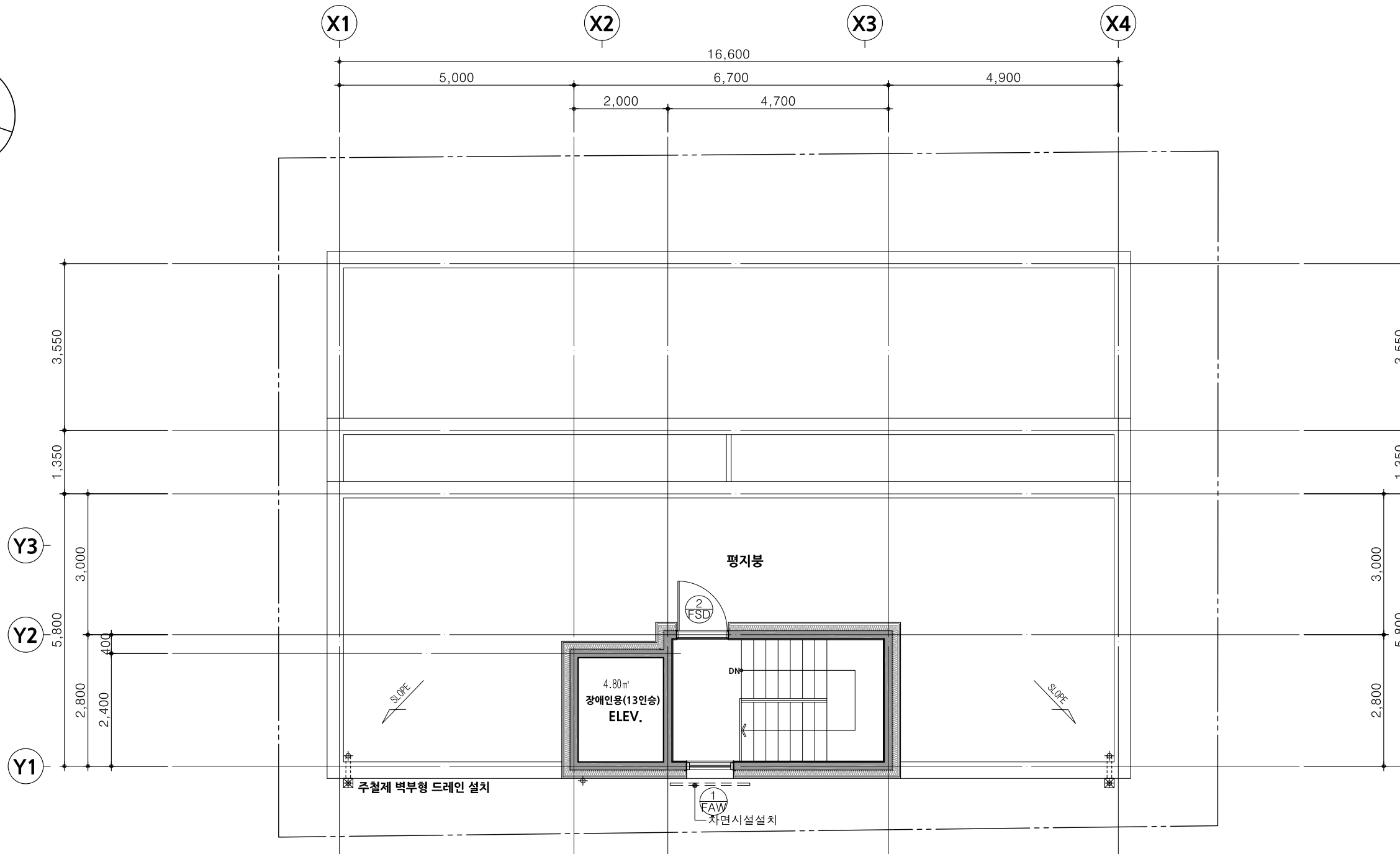
1 옥탑 평면도 축척 1:100
