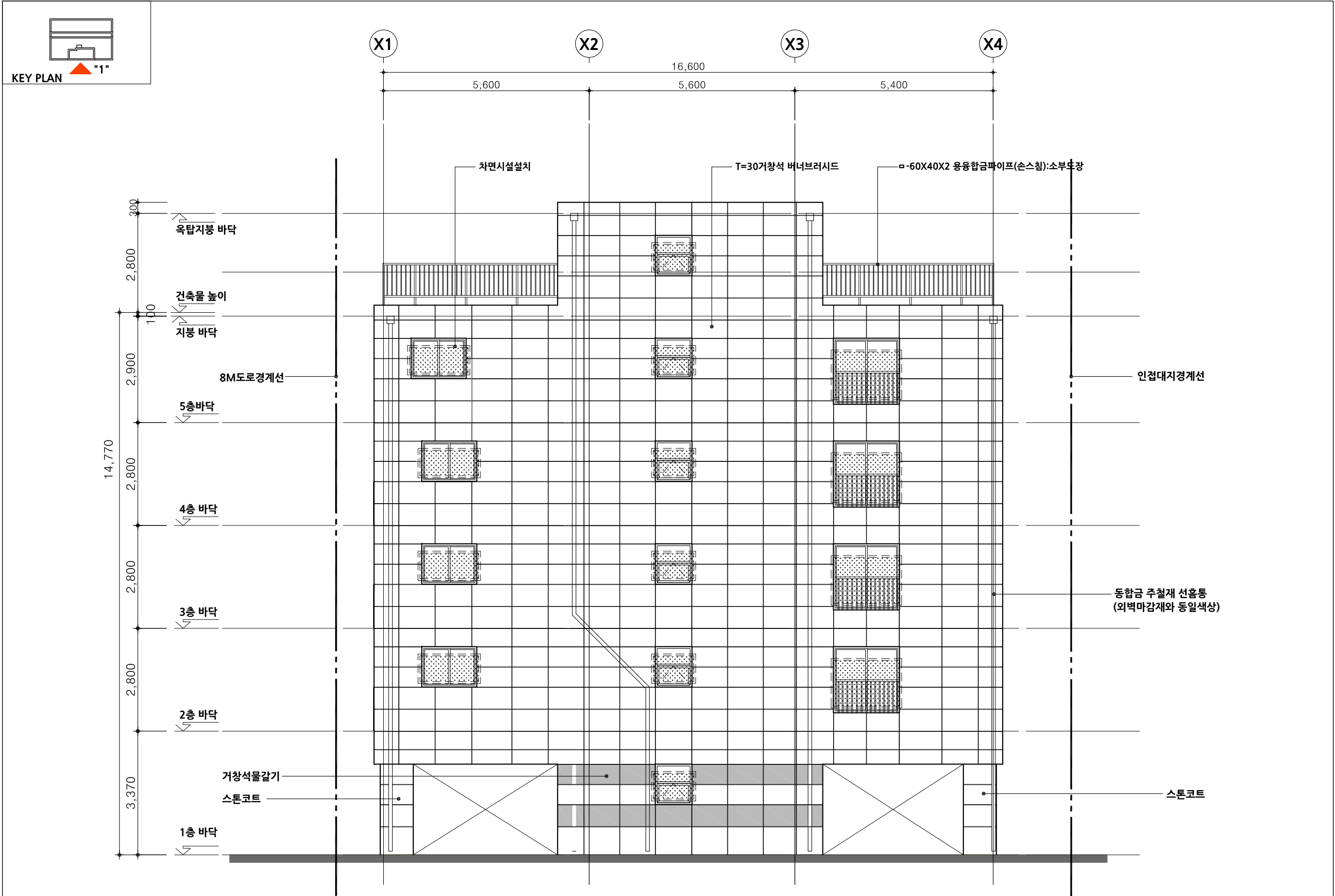
1 우측면도(남측면도) 축척 1:100
